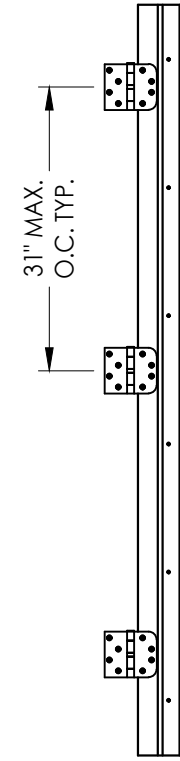
HINGE JAMB
